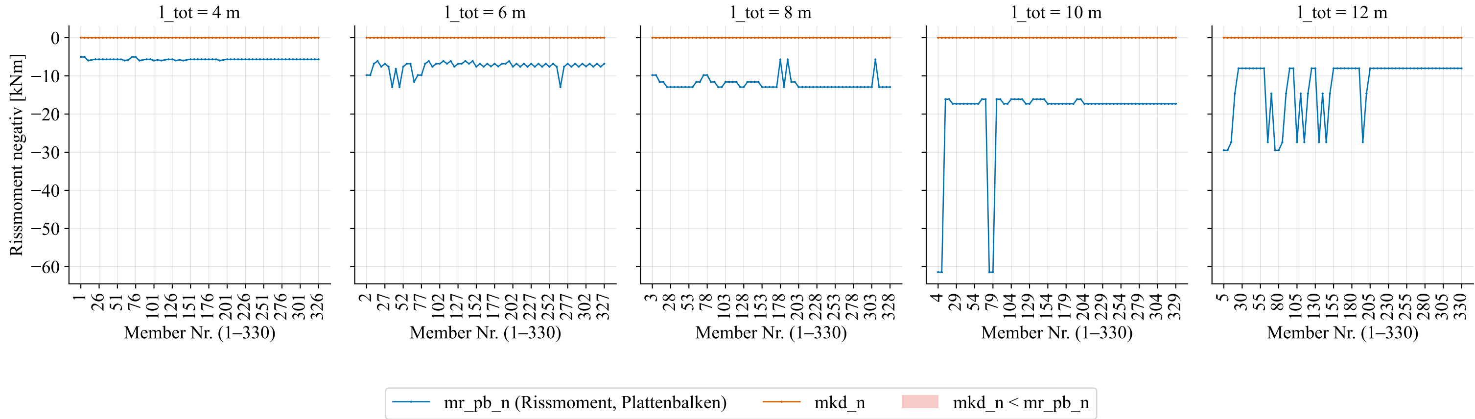
Rissmoment mr\_pb\_n (Plattenbalken) vs. Moment mkd\_n (negative Biegung) je Member, kategorisiert nach Spannweite (Members_rc_rib_simple_V3)
